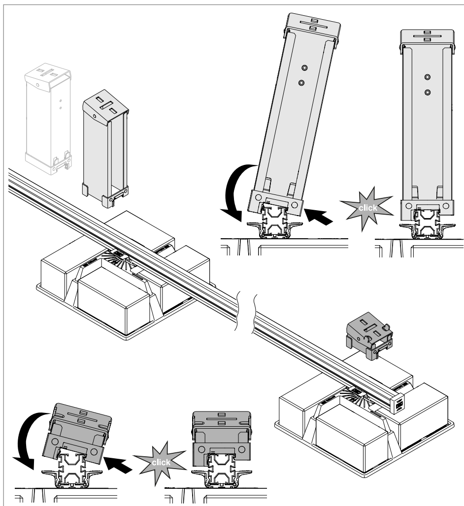
Rys. 12: Montaż podpór
