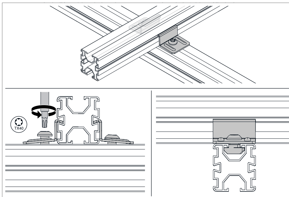
Rys. 45: Przykręcanie łącznika krzyżowego
