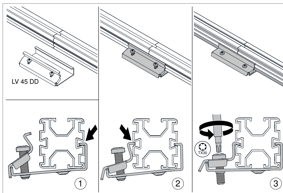
Rys. 43: Montaż łączników wzdłużnych
