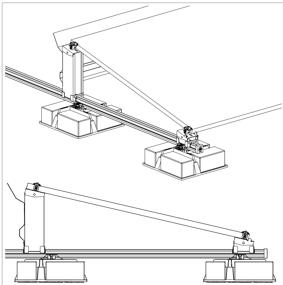
Rys. 1: Przegląd konstrukcji systemu, mocowanie boczne
