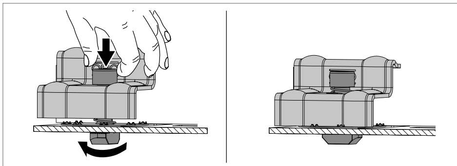
Rys. 26: Przechylenie nakrętki ślizgowej
