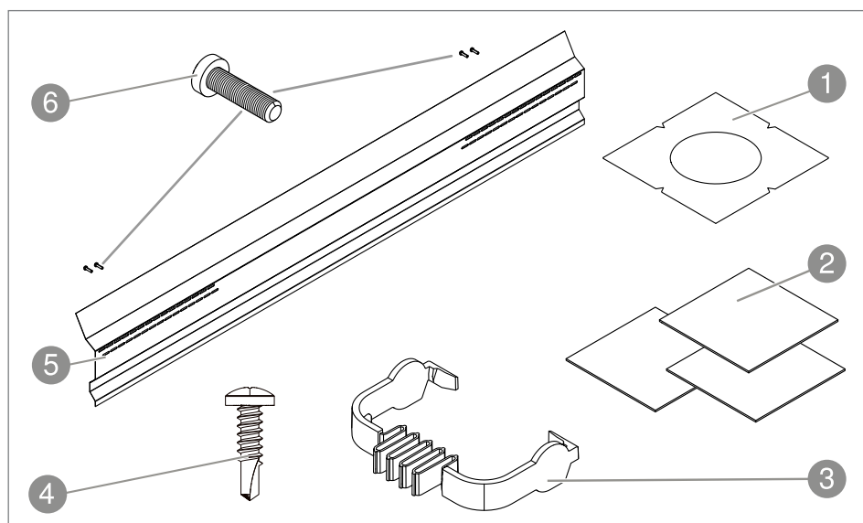
Rys. 4: Akcesoria systemowe
