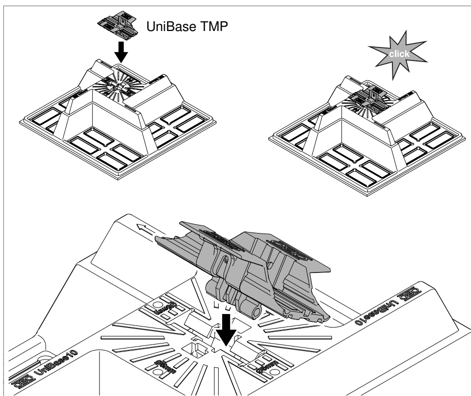
Rys. 6: Umieszczanie adaptera
