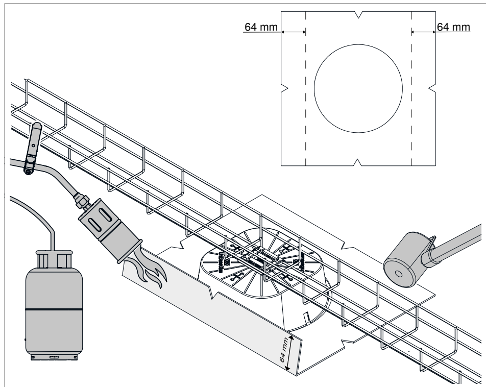
Rys. 51: Zgrzewanie mankietu
