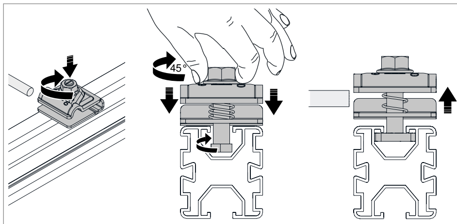
Rys. 41: Przechylenie śruby z łbem młoteczkowym w profilu nośnym
