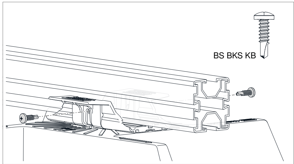
Rys. 9: Zabezpieczanie profilu nośnego śrubami
