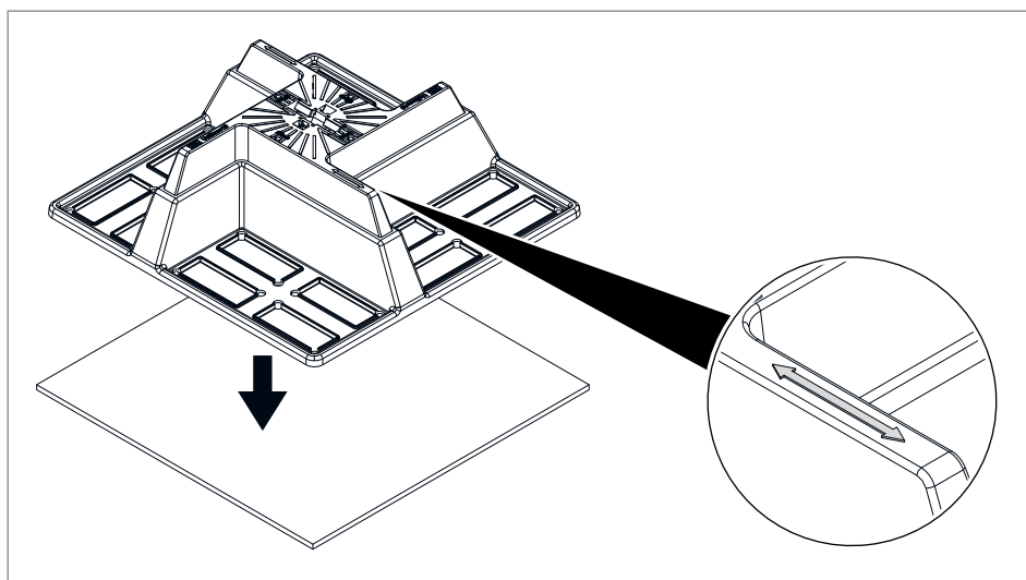
Rys. 5: Ustawianie podstawy
