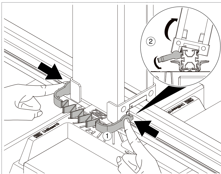
Rys. 53: Zdejmowanie podpór
