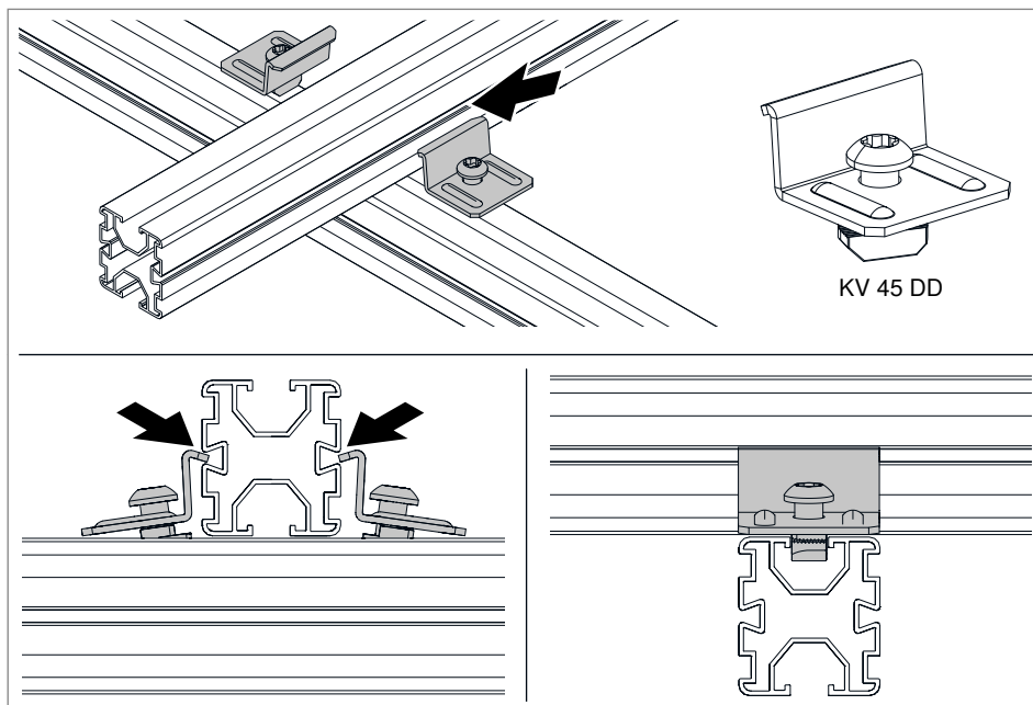
Rys. 44: Umieszczanie łącznika krzyżowego
